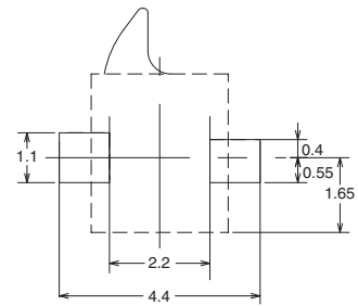
印刷基板焊盘尺寸图 (参考) (TOP VIEW)
