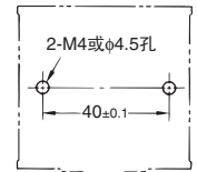
安装孔加工尺寸
