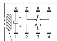
端子配置/内部连接图 (BOTTOM VIEW)
